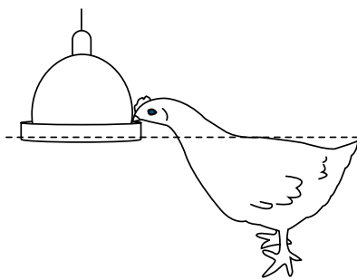
Рис. 2.4: Высота колокольной поилки
