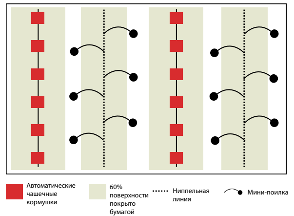
Рис 1.6: Типичное устройство птичника при использовании всего помещения в брудерный период
