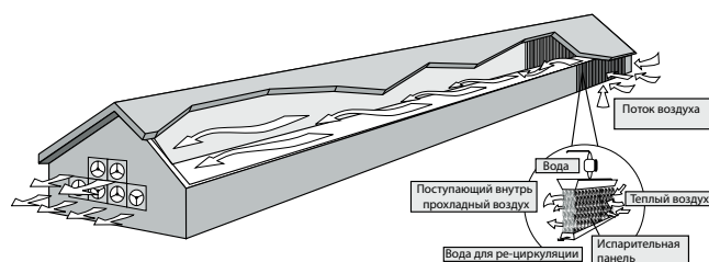
Рис. 4.4: Охлаждение с помощью испарительных панелей и туннельной вентиляции
