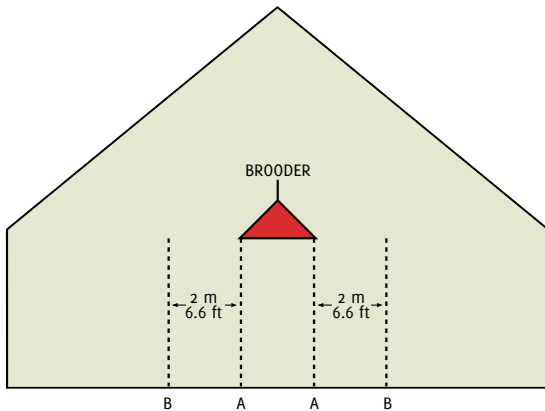
Рис 1.3: Точечный брудер – температурные зоны
