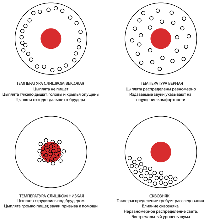
Рис 1.4: Расположение цыплят под брудером
