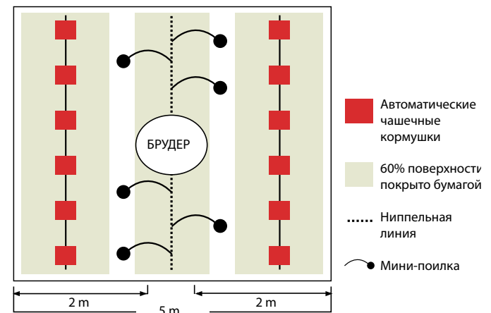
Рис 1.2: Типичное размещение точечного брудера (на 1000 цыплят)
